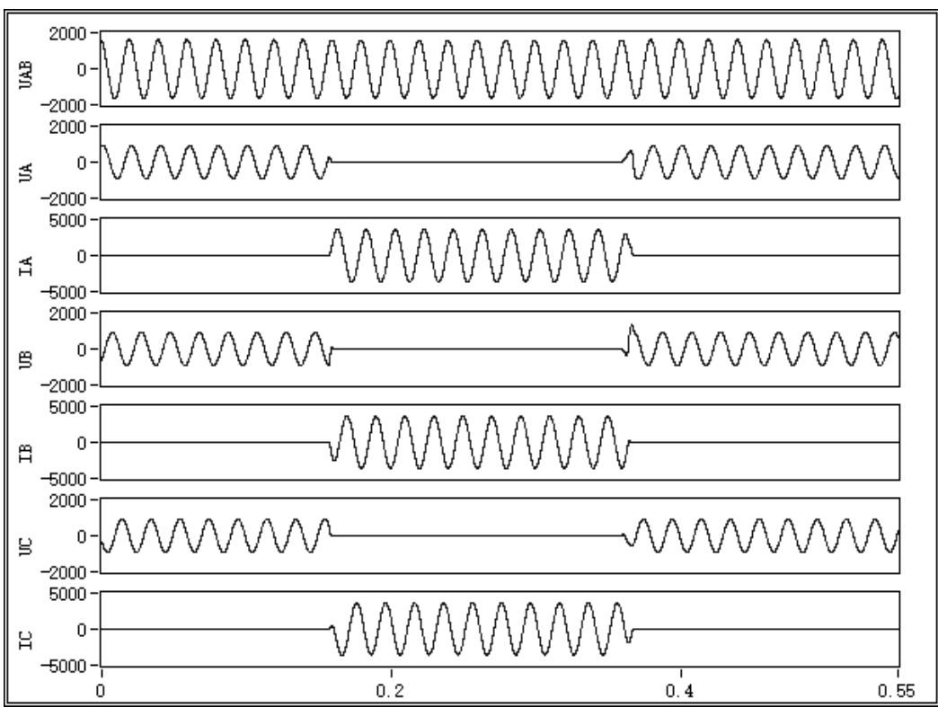
试 验 示 波 图
